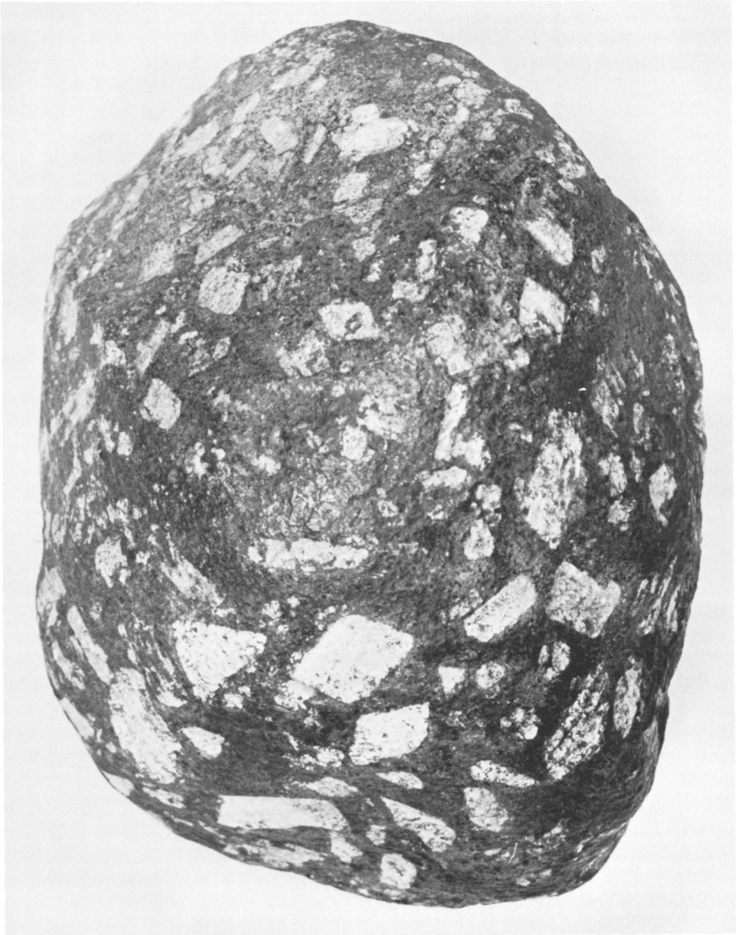
Afb. 1. Rhombenporfierdiabaas van Herikerberg No. 1545. Halve ware grootte 20 x 27 x 20 cm, 11,5 kg. Totaal aanzicht bovenzijde.
