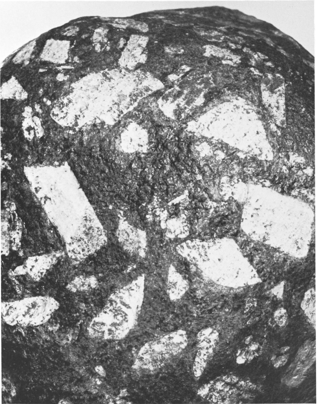
Afb. 2. Rhombenporfierdiabaas van Herikerberg No. 1545. Ware grootte 20 x 27 x 20 cm, 11,5 kg. Detail bovenzijde.
