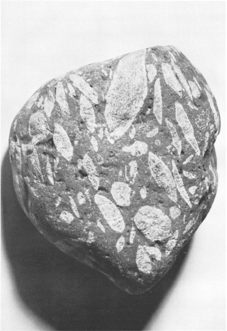
Afb. 3. Rhombenporfier van Rolde No. 84 Vrijman. 2x ware grootte. 5 x 7 x 8 cm ca. 700 gr.
