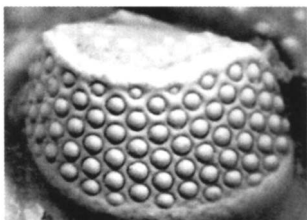
Afb. 5. Schizochroaal oog (uit Levi-Setti 1993). Afgebeeld is het oog van Phacops latifrons .
