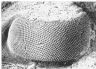
Afb. 3. Holochroaal oog (uit Clarkson 1975). Afgebeeld is het oog van Paralejurus brongniarti
