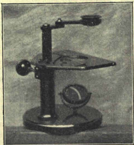
Statief met loupen (Prepareermicroscop).
