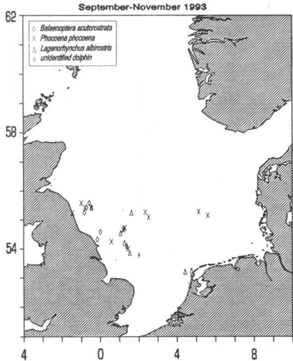
Figuur 2. Waarnemingen van walvisachtigen, sep-nov 1993. Figure 2. Sightings of cetaceans, Sep-Nov 1993.
