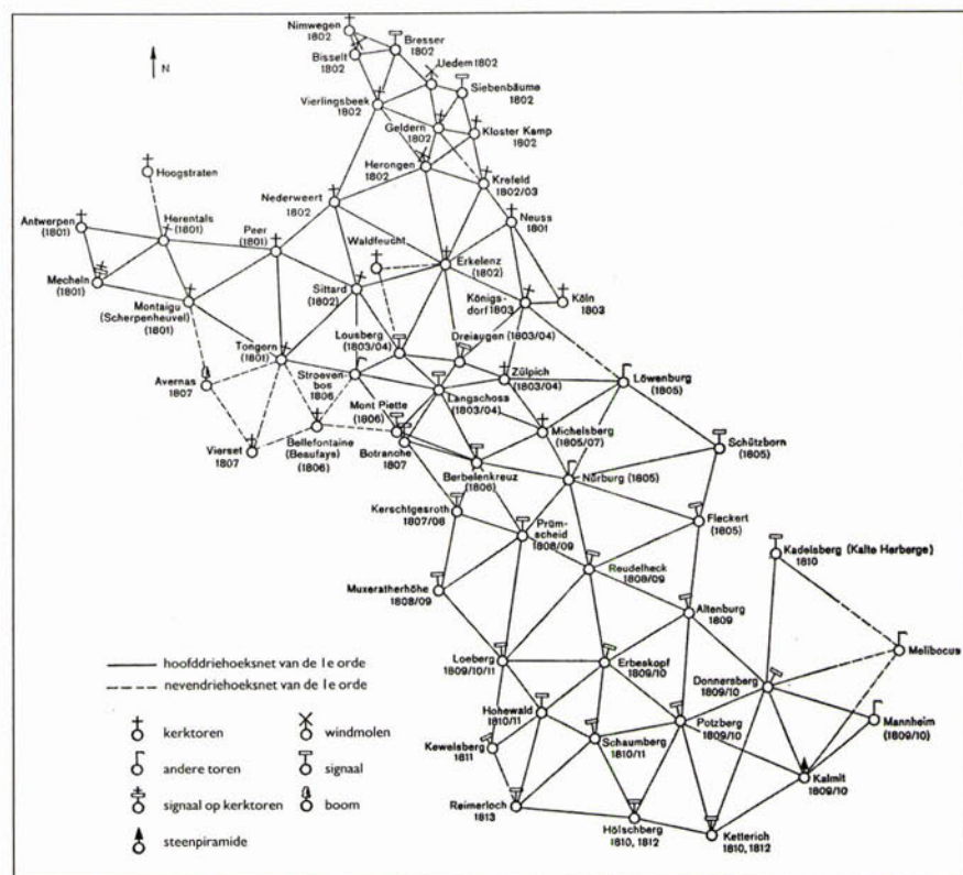
FIGUUR 7. Driehoeksnets van de 1e orde over de Franse Vier Verenigde Departementen, vervaardigd door Tranchot in de periode 1801-1810. De jaartallen bij de oriëntatiepunten hebben betrekking op de observatiejaren (uit SCHMIDT, 1973).
