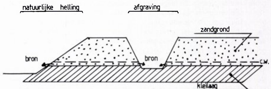
Figuur 2. Schematische voorstelling van de waterhuishoudkundige situatie binnen de overgangszone (uit eindplan ontgronding Maalbeek).
