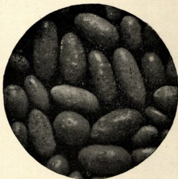
Coprolithen uit de Kunrader formatie (K). 20×ver groot.
