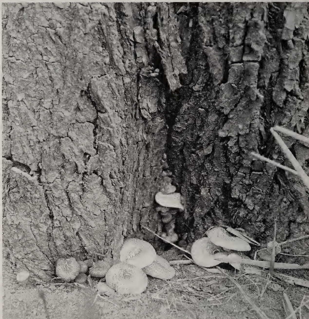
Fig. 1. Lentinus tigrinus , de tijgertaapijlat. Uit deze bundel paddestoelen werd een vrouwtje van Lordithon pulchellus verzameld.
