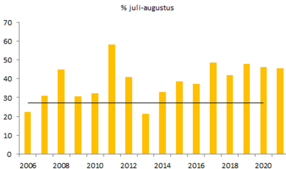
Figuur 1. Aandeel (%) per jaar in juli en augustus gestrande bruinvissen ten opzichte van het jaartotaal voor het hele land. Om een vergelijking met 2021 te kunnen maken, zijn voor alle jaren alleen de aantallen tot en met 31 augustus meegenomen. De lijn geeft het gemiddelde over 2006-2020.
