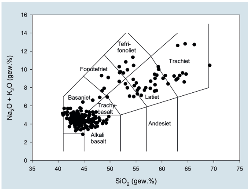
AFBEELDING 2. | Totaal alkali-silica (TAS)-diagram voor de classificatie van magmatische gesteenten met daarin geplotted gesteenten uit het Zevengebergte (data van Kolb et al., 2012 en referenties daarin).
