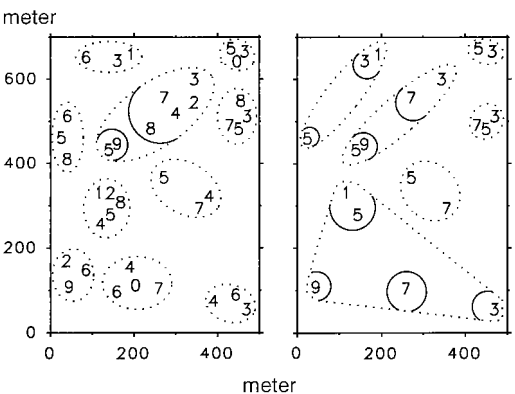
Figuur 1. Analyse van een soortkaart (Koolmees) met BMP-criteria leidt tot tien territoria na tien bezoeken (tk 0.38), of zes territoria (tk 0.63) als vijf (oneven) bezoeken gebruikt worden (....). Interpretatie met BMP-criteria en limiet aan de territoriumdiameter (200 m, —) geeft bij tien en vijf bezoeken elf territoria en dezelfde trefkans (0.35). Bezoeken 3 tot en met 9 waren in geldige periode. Aanduidingen van uitsluitende waarnemingen werden weggelaten. Analysis of a species map (Great Tit) yields ten (ten visits) or six (five visits, uneven, observed registration efficiencies 0.38 and 0.63) territories when BMP guidelines are applied (....). Limiting the territory diameter (200 m, —) yields eleven territories (registration efficiency 0.35) after both ten and five visits. Visits 3 through 9 were in the valid period.
