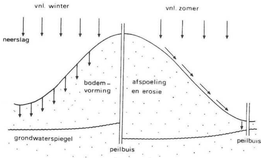
Fig. 1. Doorsnede door een duin. De pijlen geven de waterbeweging aan.
