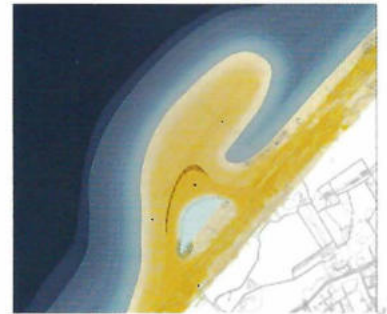
Welke invloed zullen getijde, golven, wind en recreanten hebben op het schiereiland dat tussen Kijkduin en Ter Heijde wordt aangelegd? Een interessant experiment is het in elk geval. Afbeelding: www.kustvisie.nl/zandmotor .
