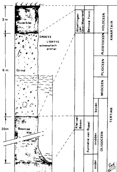
Fig.2. Lithologisch profiel groeve L'Ortye Ontsluiting 59H - 11 bij Beek.
