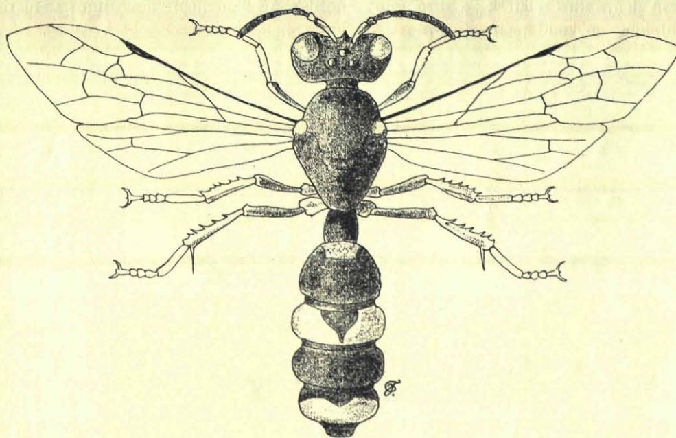
De graafbij-dooder. ( Cerceris ornata , \times 5 ).
