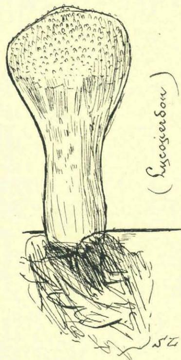
Stuifbal.
