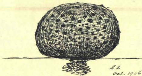
Stuifbal ( Scleroderma ).
