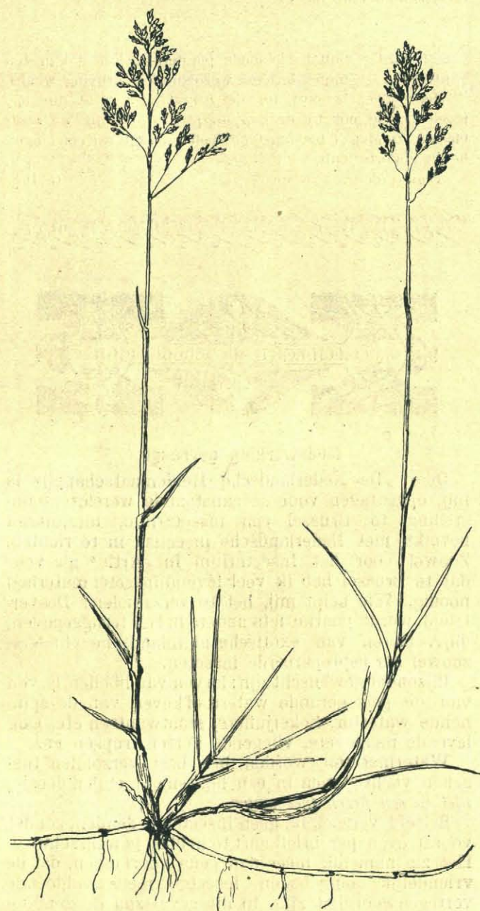
Poa pratensis L. var. costata Hartm.
