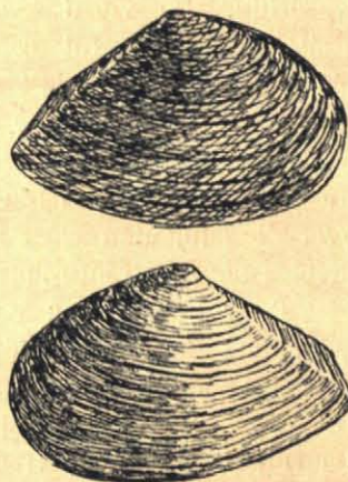
Fig. 1. Tellina fabula .
