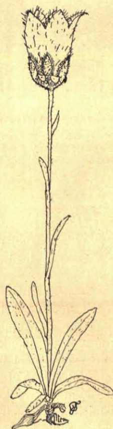
Baardklokje, rechtop.
