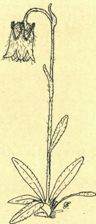
Baardklokje, gewoon.
