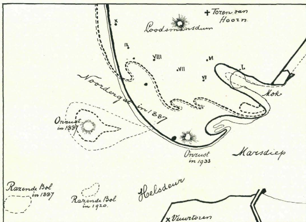
Fig. 1. De zware stippellijn is de hoogwaterlijn in 1887, de lichte stippellijn de laagwaterlijn in hetzelfde jaar. De zware doorgetrokken lijn is de hoogwaterlijn in 1931, de lichte lijn de laagwaterlijn in hetzelfde jaar.
