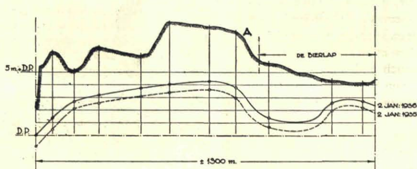
Fig. 5. Grafiek grondwater. De grillige grondwaterlijn sterk afwijkend van het gewone schema. Uit: „Onze Duinen”.
