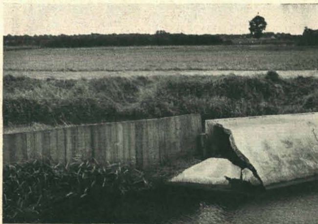
Fig. 4. De instortingsplaats met de houten damwand.
