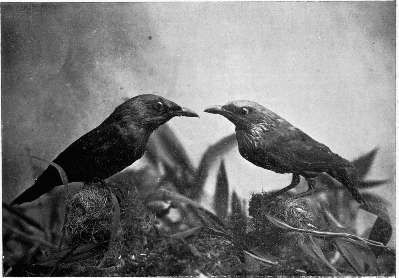
Fig. 3. Calornis chalybea .
