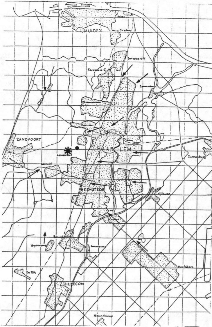
Figuur 1. Kaart van Zuid-Kennemerland met slaapplaats van Zwarte Kraaien (ster), voorverzamelplaats (stip) en waargenomen vlieg-richtingen 's avonds (pijlen).
