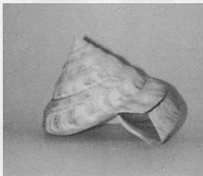
het holotype van Pleurotomaria rumphii Schepman 1879 (coll NMR no 13873)
