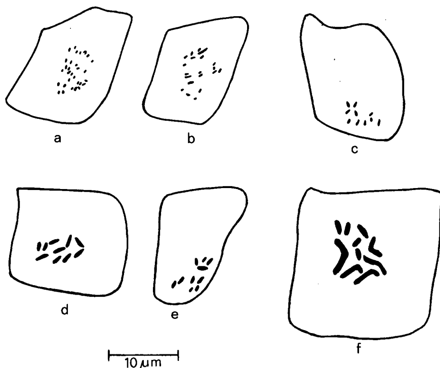
Fig. 2. Karyograms of the investigated species (schematic). a. Riccardia chamedrifolia (Kortenhoeft); b. R. multifida (Kortenhoeft); c. R. incurvata (Staverden); d. R. incurvata (Venlo); e. R. incurvata (Schiermonnikoog); f. Aneura pinguis (Wassenaar).
