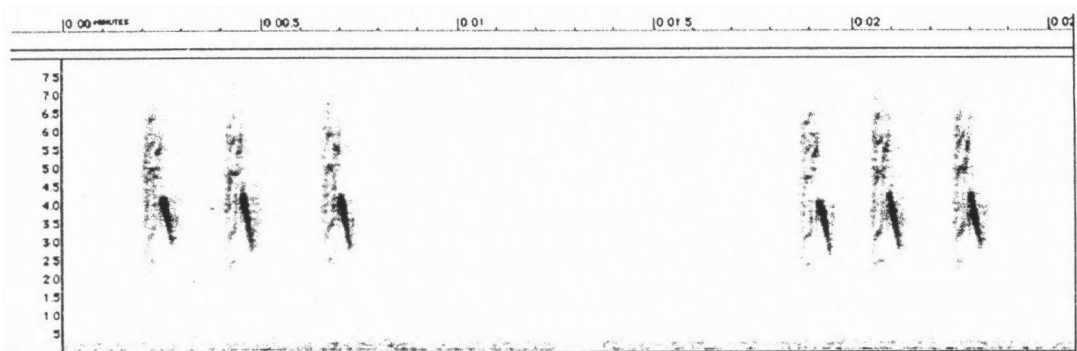
Figuur 1. Roep Noordafrikaanse Vink, Marokko. Opname Arnoud van den Berg. Sonogram Magnus Robb. Print Rik Winters.
