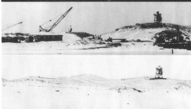
Duinkruising Callantssoog, situatie tijdens en na het leggen van de pijpleiding.
