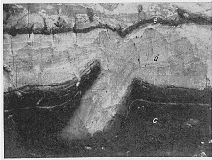
Abb. 4. Spätglazialer kryoturbater Torf (organogene Ablagerung c ) unter spätglazialem Decksand (aeolische Ablagerung d ) mit humoser Schicht (organogen-aeolische Ablagerung e ). Dicke der humosen Schicht \pm 4 cm. Kanalwand Wiene 1937.
