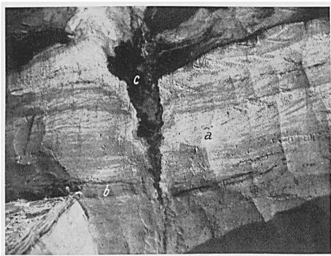
Abb. 5. Würm-stadialer Sand (aquatile Ablagerung a ) mit Dryasfloraschicht b ) und spätglazialem kryoturbatem Torf (organogene Ablagerung c ). Dicke der Dryasfloraschicht \pm 5 cm. Kanalwand Wiene 1937.
