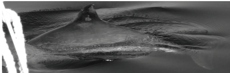
Figuur 10. Rug en linkerflank van Bruinvis meezwemmend met zeiljacht, 28 september 2008. - Left side of bowriding Harbour Porpoise near yacht, 28 September 2008 (Karin Heijboer).
