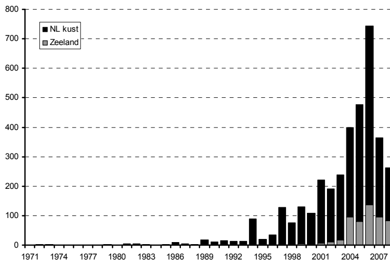
Figuur 1. Gerapporteerde waarnemingen van Bruinvissen langs de Nederlandse Noordzeekust ( >52^{\circ}N ; zwart, 3048 sightings) en in Zeeland (grijs, 546 sightings) sinds 1970. - Reported sightings per annum of Harbour Porpoises along the North Sea coast (black, 3048 sightings) and in Zeeland (grey, 546 sightings) (Marine Mammal Database).
