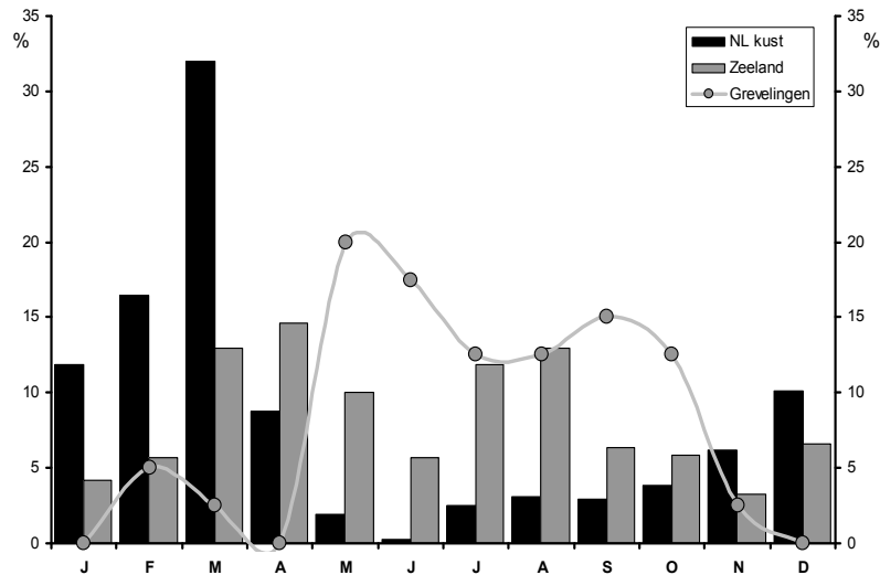
Figuur 2. Seizoenpatroon van gerapporteerde waarnemingen van Bruinvissen langs de Nederlandse Noordzeekust (>52°N; zwart), in Zeeland (grijs) en in het Grevelingenmeer (lijn). - Seasonal pattern in reported sightings of Harbour Porpoises along the North Sea coast (black), in Zeeland (grey) and in Lake Grevelingen (line) (Marine Mammal Database).
