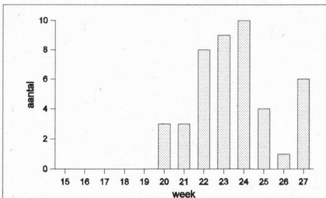
Figuur 2. Verdeling van de aantallen Kwartelwaarnemingen in 1997 over de inventarisatieperiode (tweede week april tot eerste week juli) van het Weidevogelmeetnet Friesland.
