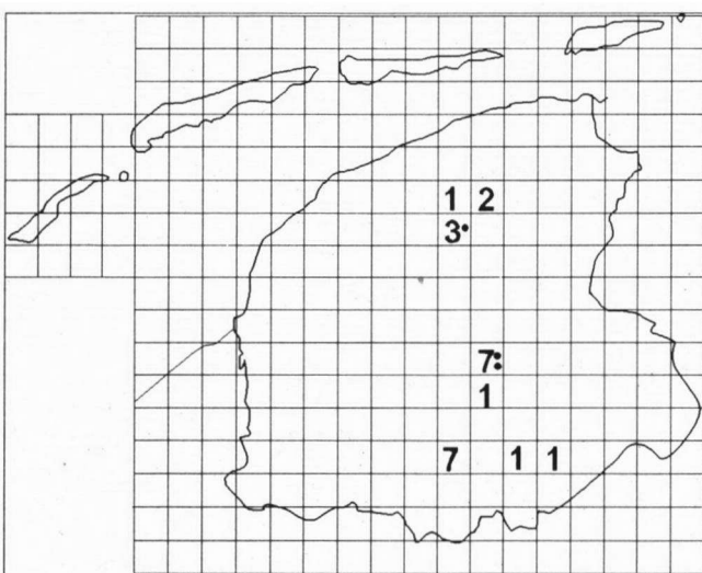
Figuur 1. Territoria van de Kwartel (23) en de Kwartelkoning (3), vastgesteld in proefvlakken (50) van het Weidevogelmeetnet Friesland in 1997. De getallen geven de aantallen Kwartel-territoria per atlasblok. Territoria van de Kwartelkoning zijn weergegeven door een stip.
