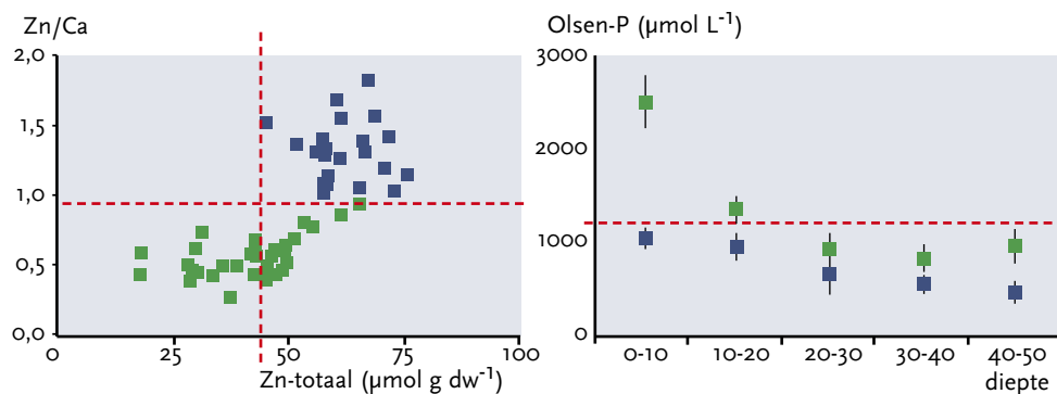
Fig. 1. Totaal Zn-gehalte, Zn/Ca-ratio van de bodem en de hoeveelheid plantbeschikbaar fosfaat (Olsen-P) op locaties in stroomdalgraslanden langs de Geul waar zinkvegetatie nog voorkomt en waar deze de afgelopen decennia verdwenen is (uit: Lucassen et al., 2008).
