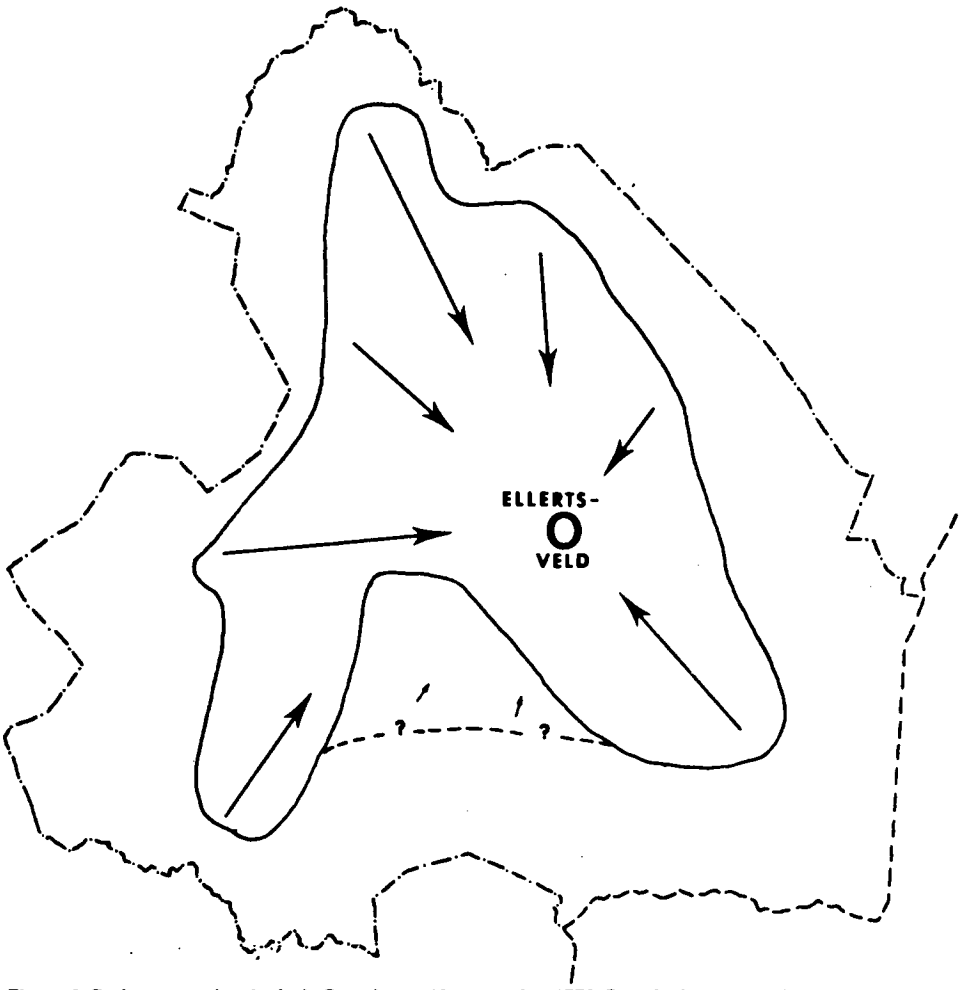
Figuur 6. De laatste wolvenjacht in Drenthe op 19 september 1772. Deze jacht was zonder succes. Te Dwingeloo werd wel een Wolf gezien. Naar gegevens van Oltmans (1906).
