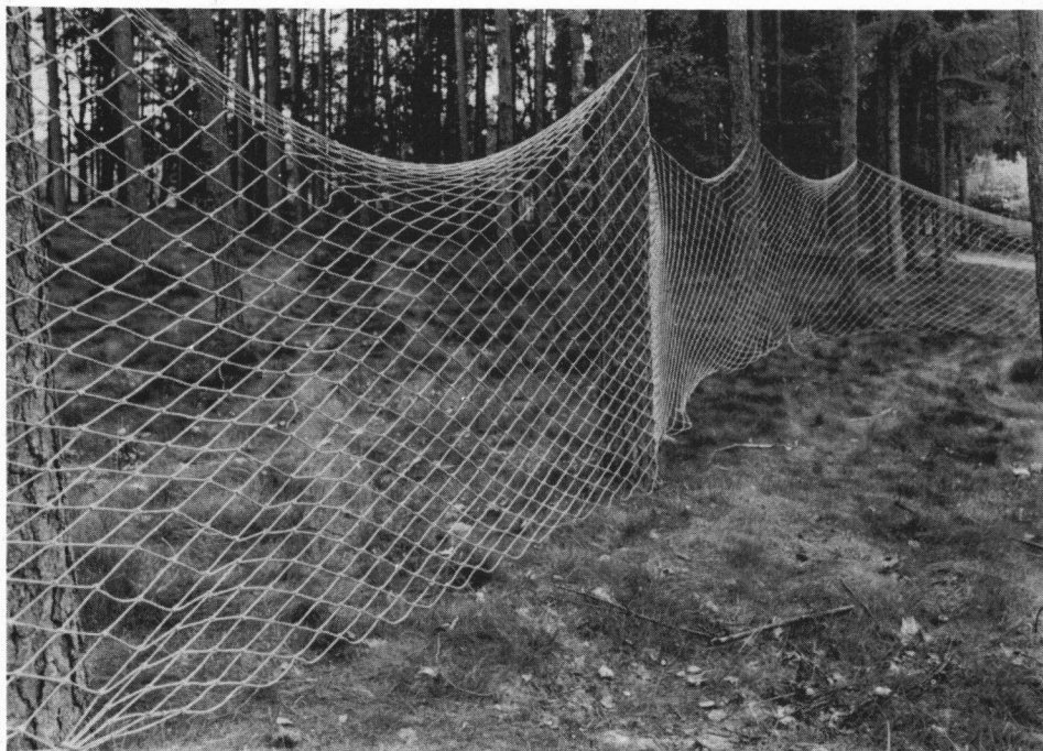
Figuur 8. Het wolvennet uit de kerk van Cuyk. Foto: Nederlands Openluchtmuseum, Arnhem.
