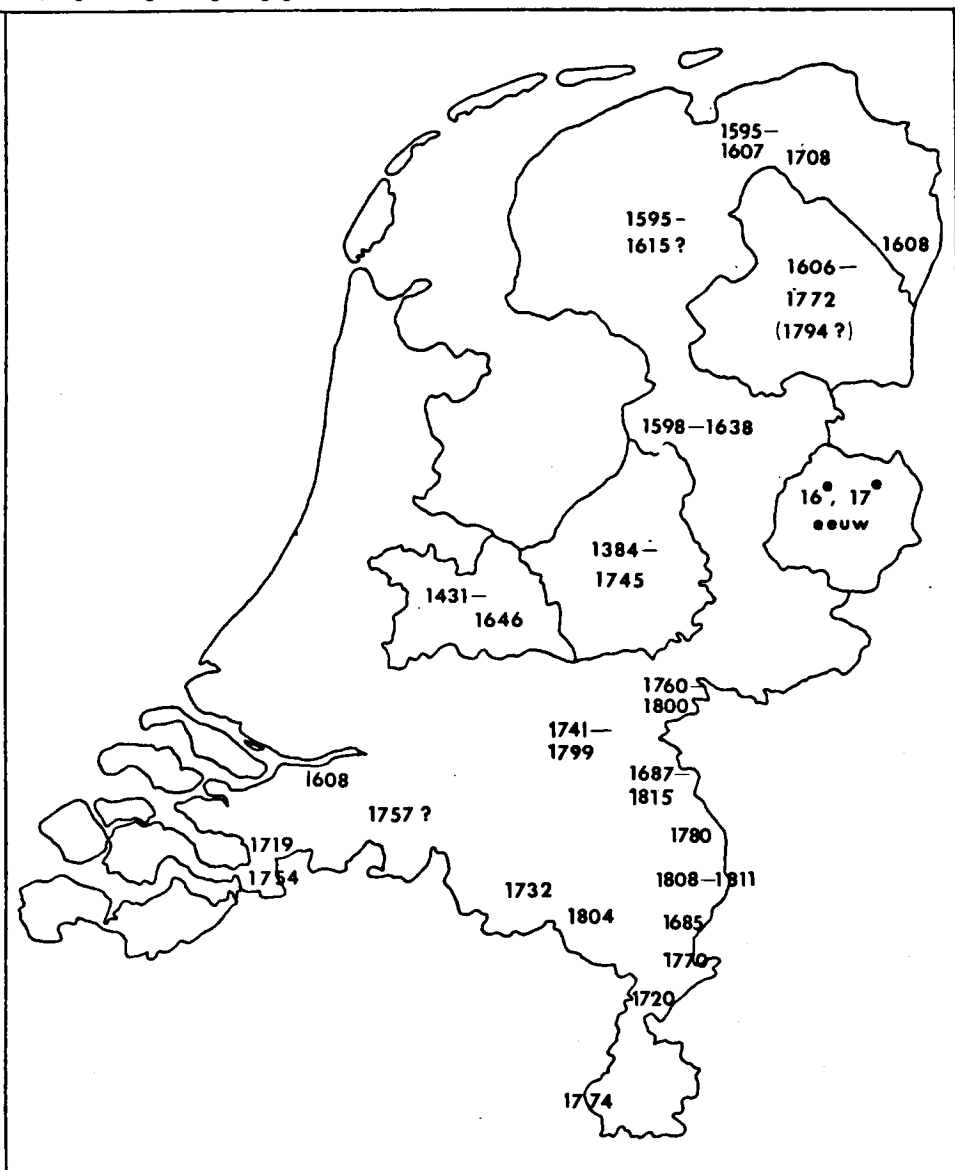
Figuur 2. Wolvenjachten in Nederland. Per streek is het eerste en laatste jaar vermeld, waarin een wolvenjacht werd gehouden. Bij kleine wolvenjachten en bij jachten waarvan onbekend is welk gebied ze omspannen, is geen begrenzing aangegeven.
