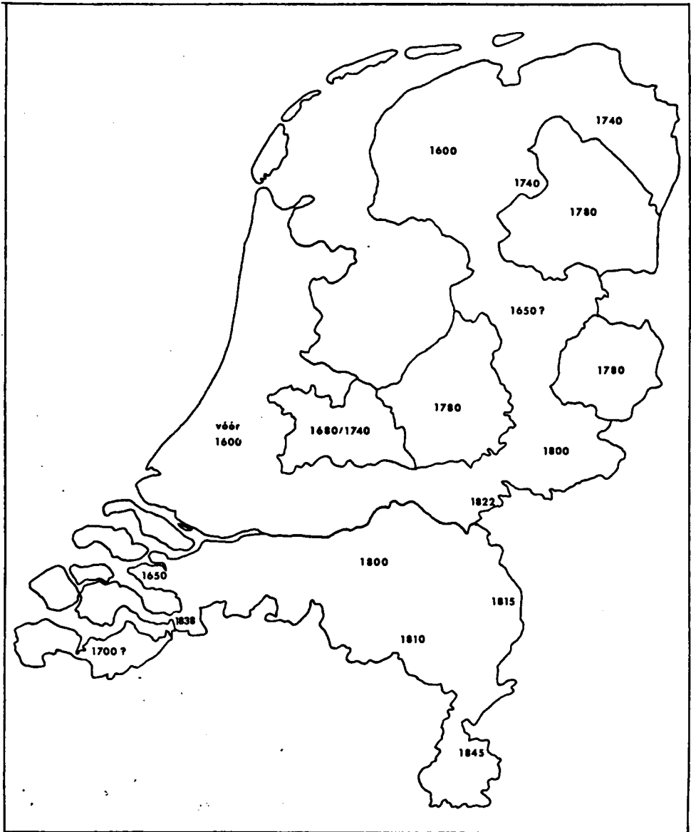
Figuur 1. Afname in de verspreiding van de Wolf. Het jaar waarin de laatste Wolf in een gebied werd waargenomen is aangegeven. Voor Utrecht worden in de literatuur twee zeer uiteenlopende jaren genoemd, die daarom maar beide zijn opgenomen.
