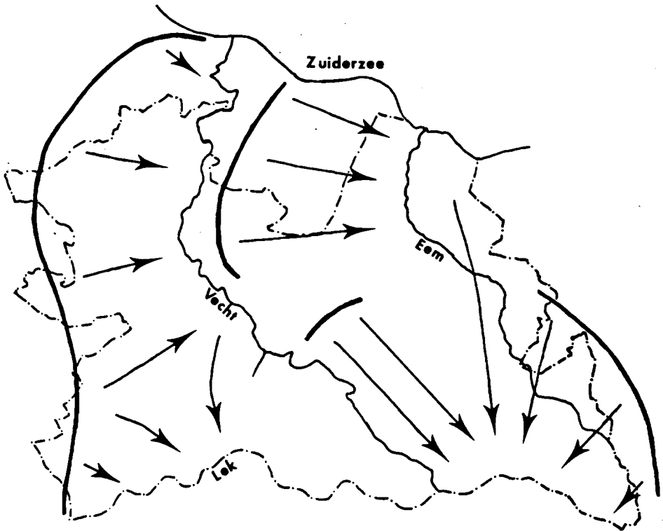
Figuur 3. Wolvenjacht in Utrecht op 14 april 1592. De naar de rivieren gedreven Wolven werden daar in schuiten opgewacht. Naar gegevens van Van de Water (1729 : 414).
