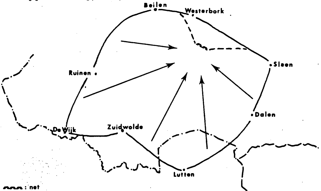
Figuur 5. Wolvenjacht in Zuid-Drenthe op 8 oktober 1618. Een paar deelnemende dorpen zijn aangegeven. Naar gegevens van Joosting (1912 : 239).
