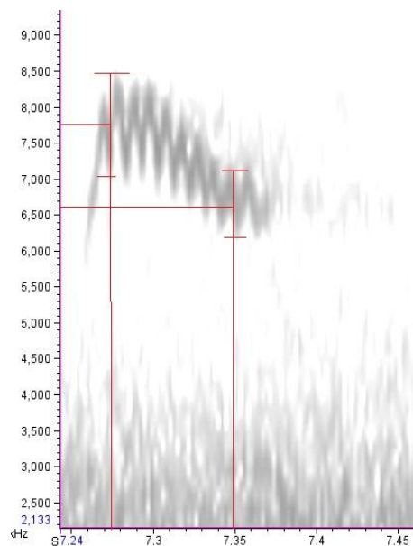
Siberische Boompieper sonogram Jacob Lotz 10-10-2016
