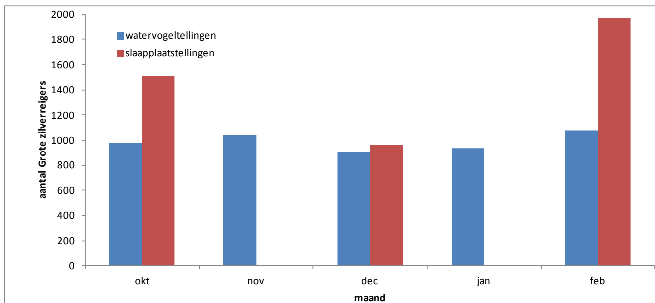
Figuur 1. Aantallen Grote zilverreigers in Fryslân in de winter van 2014/2015 tijdens maandelijkse watervogeltellingen en op slaapplaatsen in oktober, december en februari..
