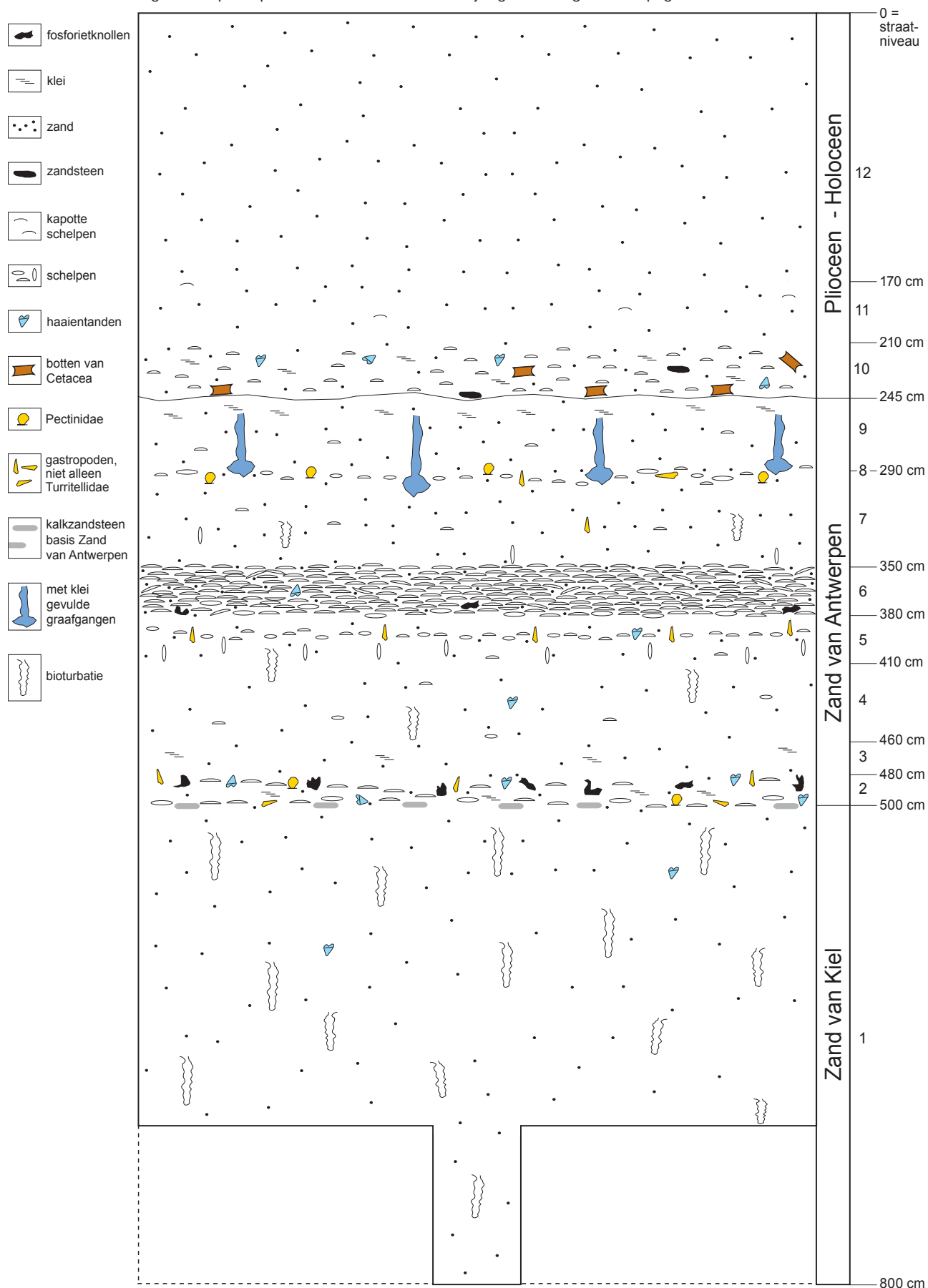
Fig. 5: Composietprofiel van PHB-2. Voor beschrijving van de lagen zie de pagina's 68-73.
