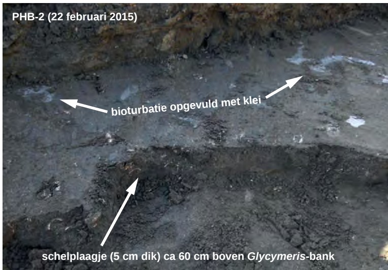
Fig. 11: PHB-2. Schelpplaagje ca 60 cm boven de Glycymeris -bank, met bioturbatie (graafgangen).
