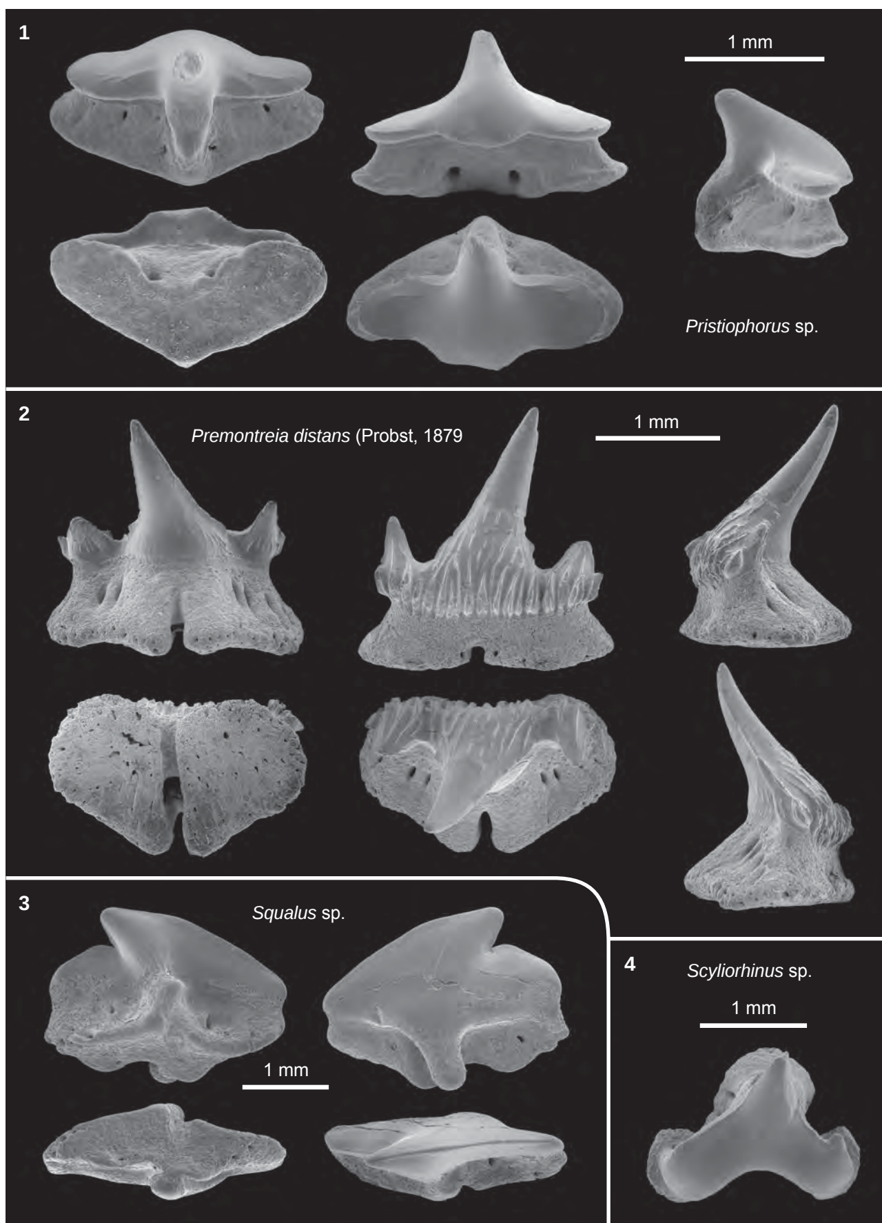
Plaat 1: Enkele haaiantanden uit het schelpplaagje ca 60 cm boven de Glycymeris -bank, Zand van Antwerpen. 1. Pristiophorus sp. 2. Premontreia distans (Probst, 1879). 3. Squalus sp. 4. Scyliorhinus sp.
