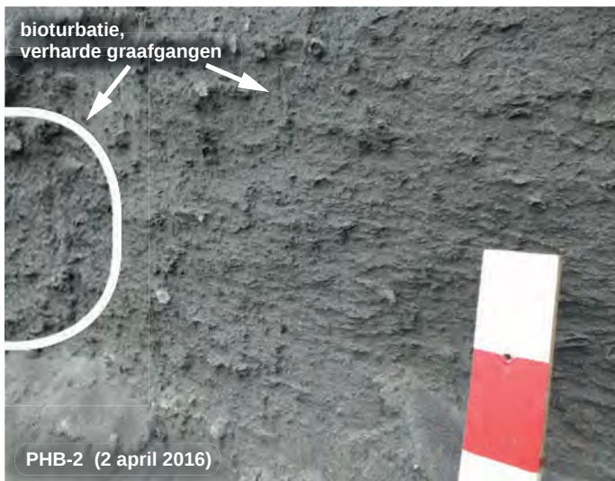
Fig. 6: PHB-2. Bioturbatie in Zand van Kiel, foto genomen op 2 april 2016 na enkele dagen van regen en felle wind, die het zand tussen de graafgangen wegblies. (Links in kader een verharde graafgang in detail.)
