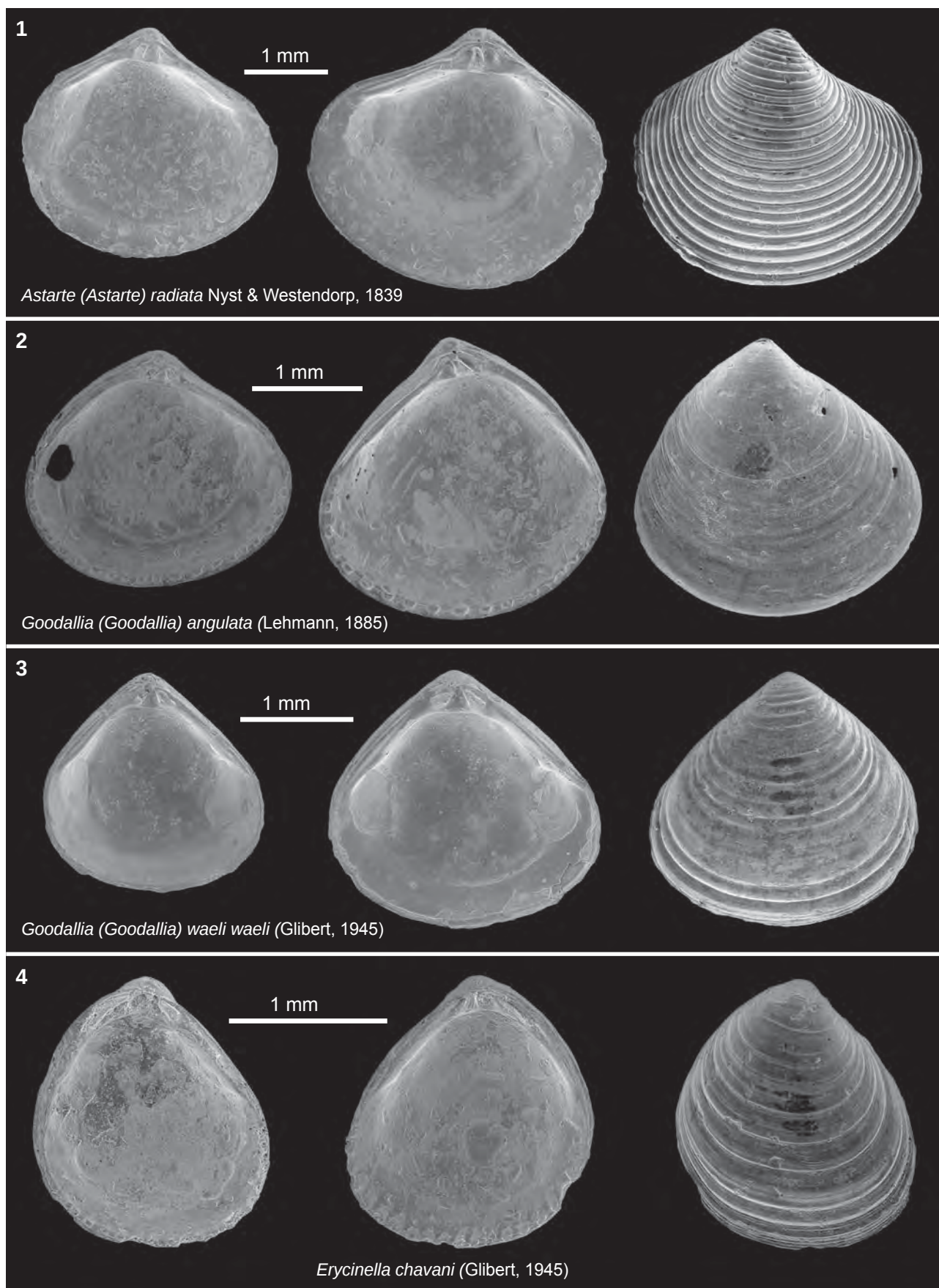
Plaat 3: Enkele mollusken uit het schelpplagje ca 60 cm boven de Glycymeris -bank, Zand van Antwerpen. 1. Astarte (Astarte) radiata Nyst & Westendorp, 1839. 2. Goodallia (Goodallia) angulata (Lehmann, 1885). 3. Goodallia (Goodallia) waeli waeli (Glibert, 1945). 4. Erycinella chavani (Glibert, 1945).
