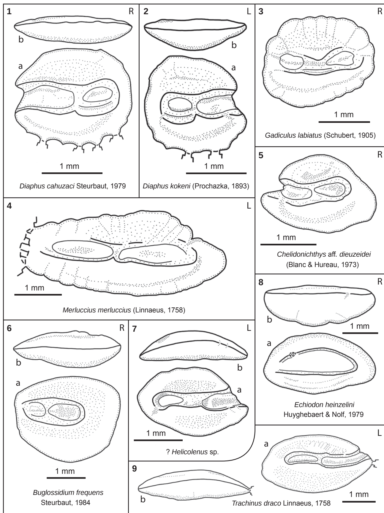
Plaat 2: Enkele otolieten uit het schelpplagje ca 60 cm boven de Glycymeris -bank, Zand van Antwerpen. 1. Diaphus cahuzaci Steurbaut, 1979. 2. Diaphus kokeni (Prochazka, 1893). 3. Gadiculus labiatus (Schubert, 1905). 4. Merluccius merluccius (Linnaeus, 1758). 5. Chelidonichthys aff. dieuzeidei (Blanc & Hureau, 1973). 6. Buglossidium frequens Steurbaut, 1984. 7. ? Helicolenus sp. 8. Echiodon heinzlini Huyghebaert & Nolf, 1979. 9. Trachinus draco Linnaeus, 1758. (De letters in de rechter bovenhoek staan voor linker otoliet 'L' of rechter otoliet 'R').
